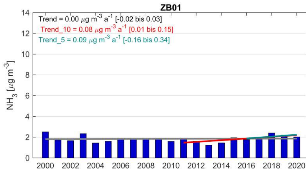
Abbildung 21: Trendberechnung der Jahresmittel am Messpunkt ZB01. In Grau ist der Trend über alle Jahre der Messperiode dargestellt, in Rot der Trend seit 2010 und in Türkis derjenige der letzten fünf Jahre.
