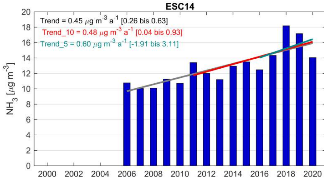
Abbildung 19: Trendberechnung der Jahresmittel am Messpunkt ESC14. In Grau ist der Trend über alle Jahre der Messperiode dargestellt, in Rot der Trend seit 2010 und in Türkis derjenige der letzten fünf Jahre. Zum besseren Verständnis wurde die y-Achsen-Skala in dieser Abbildung den Messwerten angepasst.
