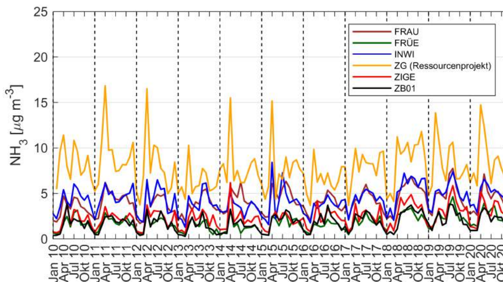
Abbildung 10: Verlauf der Ammoniakkonzentration seit Januar 2010 an den verschiedenen kantonalen Passivsammler-Standorten in Zug sowie den Zuger Ressourcenprojekt-Standorten (ZG).
