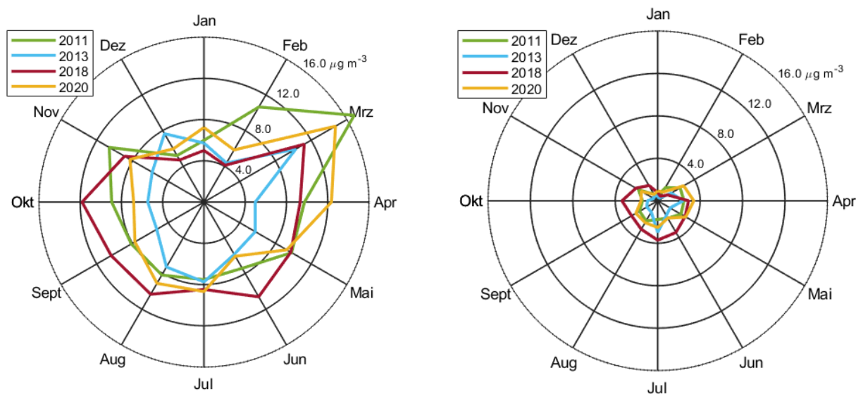
Abbildung 12: Darstellung der Monatsmittelwerte in Netzdiagrammen für das Messgebiet Zug (links) und den Messpunkt Zugerberg (rechts) für die Jahre 2011, 2013, 2018 und 2020.
