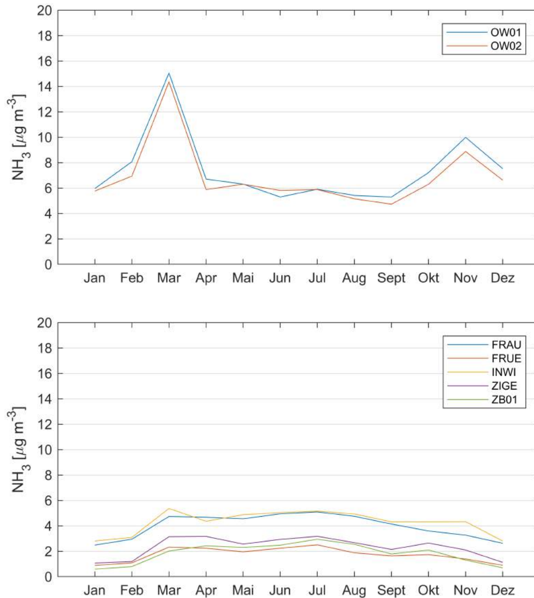
Abbildung 6: Vergleich des Jahresgangs unterschiedlicher Messpunkte mit unterschiedlicher Bewirtschaftung bzw. unterschiedlich intensiver Tierhaltung. Mittelung von 2010 bis 2020. Oben: Messpunkte von Obwalden. Unten: Messpunkte des Kantons Zug.
