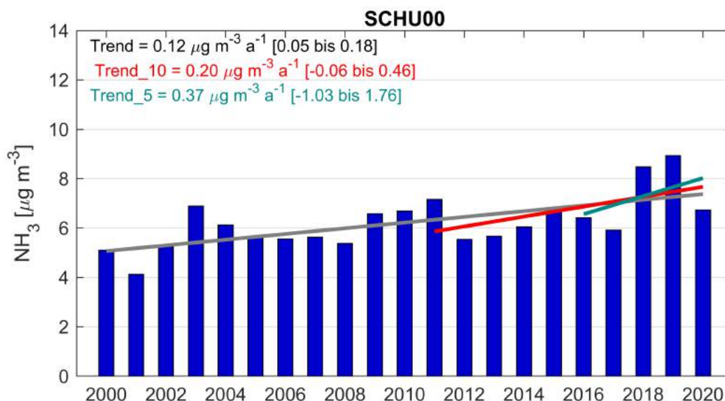
Abbildung 18: Trendberechnung der Jahresmittel am Messpunkt SCHU00. In Grau ist der Trend über alle Jahre der Messperiode dargestellt, in Rot der Trend seit 2010 und in Türkis derjenige der letzten fünf Jahre.
