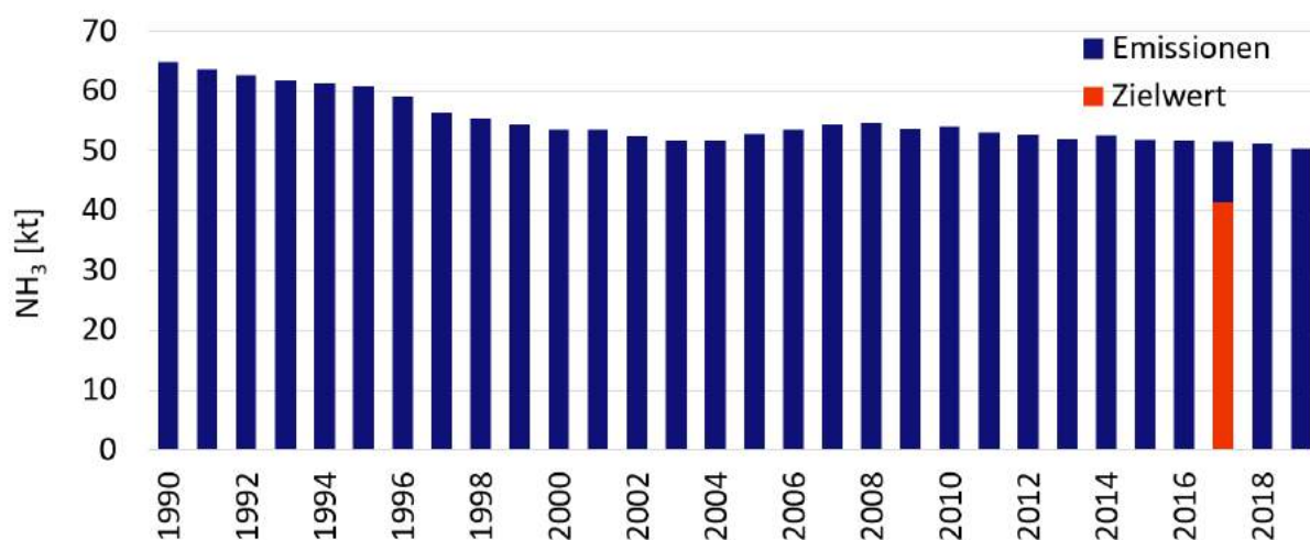
Abbildung 1: Ammoniakemissionen aus der Landwirtschaft in der Schweiz von 1990 bis 2019. 5 Der rote Balken zeigt den vom BAFU kommunizierten Zielwert für 2017.
