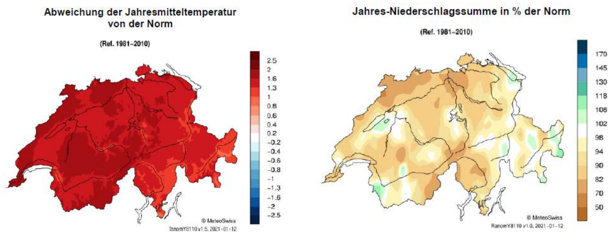
Abbildung 25: Links: Abweichung der Jahresmitteltemperatur 2020 von der Norm (1981-2010) in °C . Rechts: Jahres-Niederschlagssumme in Prozent der Norm (1981-2010). Quelle: MeteoSchweiz (2021). Klimabulletin 2020.
