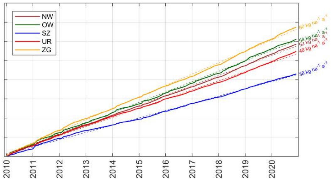
Abbildung 24: Aus gemessenen Ammoniakkonzentrationen berechnete und aufsummierte N-Deposition aller Ressourcenprojekt-Standorte der ZUDK (Ressourcenprojekt-Messpunkte seit 2010). Die gestrichelten Kurven entsprechen der linearen Regressionsfunktion. Die Zahlen am rechten Bildrand stehen für die mittleren N-Deposition durch Ammoniak pro Jahr, berechnet aus der linearen Regressionsfunktion.
