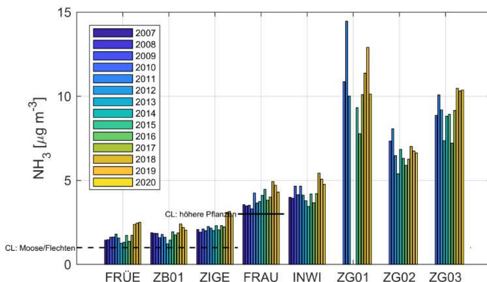
Abbildung 8: Jahresmittel (2007 bis 2020) der Ammoniakkonzentration an den einzelnen Messpunkten im Kanton Zug. Dies beinhaltet sowohl die kantonalen Messpunkte (FRÜE, ZB01, ZIGE, FRAU, INWI), wie auch diejenigen des Ressourcenprojekts (ZG0, ZG02, ZG03). Für ZG01 konnten aufgrund von Datenlücken keine gültigen Jahresmittel für 2013 und 2014 berechnet werden. Die schwarze ausgezogene Linie kennzeichnet den Critical Level (CL) für höhere Pflanzen, die schwarze gestrichelte Linie den Critical Level (CL) für empfindliche Moose und Flechten.
