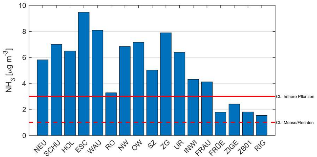
Abbildung 7: Mehrjähriges Mittel (2010 - 2020) der Ammoniakkonzentration in den einzelnen Messgebieten. Die rote ausgezogene Linie kennzeichnet den Critical Level (CL) für höhere Pflanzen, die rote gestrichelte Linie denjenigen für empfindliche Moose und Flechten.
