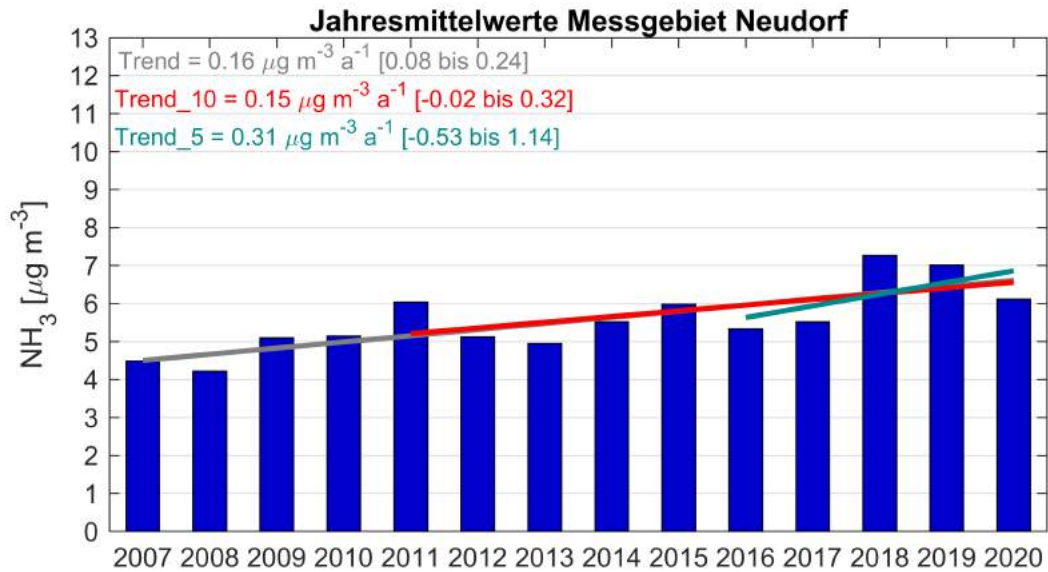
Abbildung 14: Trendberechnung für die gemittelten Jahresmittelwerte des Messgebiets Neudorf (verwendete Stationen zur Trendberechnung: NEU01, NEU02, NEU03). Der rote Trend bezieht sich auf die ganze Messperiode, der rote und türkise Trend auf die letzten zehn bzw. fünf Jahre.
