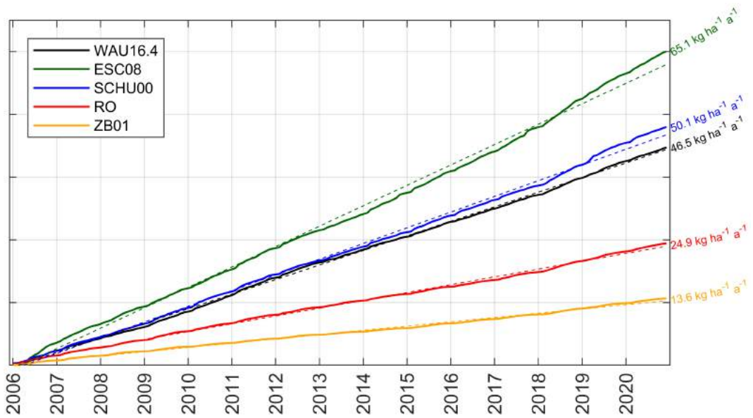
Abbildung 23: Aus gemessenen Ammoniakkonzentrationen berechnete und aufsummierte N-Depositionen seit Januar 2006 bis Dezember 2018 an fünf verschiedenen Messpunkten in der Zentralschweiz. Die gestrichelten Kurven entsprechen der linearen Regressionsfunktion, die Zahlen am rechten Bildrand stehen für die mittlere N-Deposition durch Ammoniak pro Jahr, berechnet aus der linearen Regressionsfunktion.
