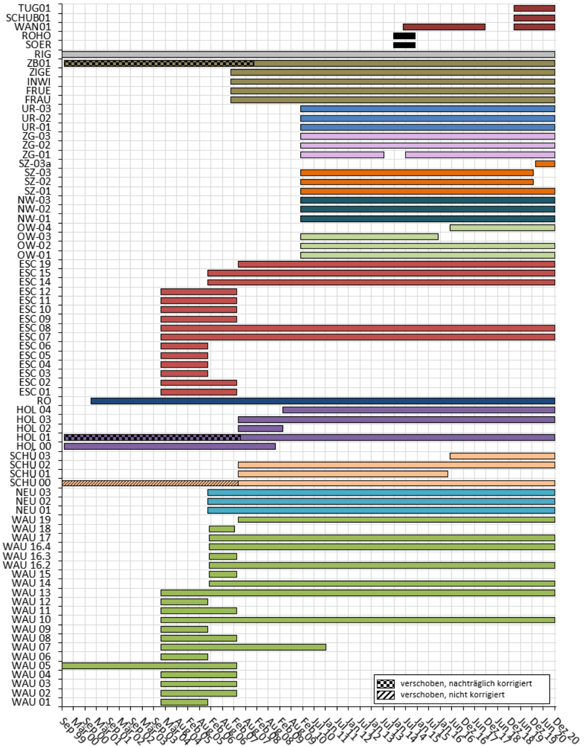
Abbildung 5: Zeitliche Übersichtstafel aller Messpunkte in der Zentralschweiz, farblich unterteilt in die verschiedenen Messgebiete.). 23
