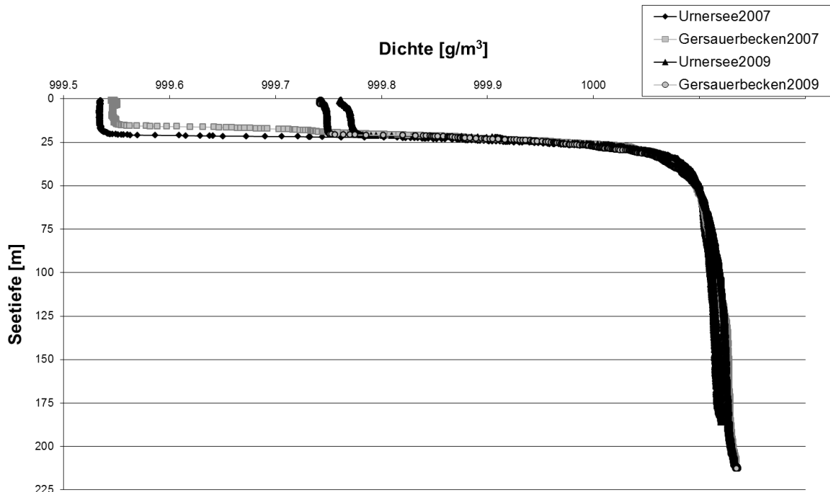
Abbildung 6: Dichtemessungen im Urnersee und im Gersauerbecken. Daten: Aufsichtskommission Vierwaldstättersee, 2010.
