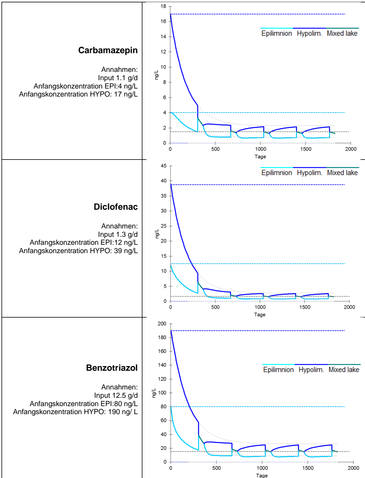
Abbildung 16: Modellierter Konzentrationsverlauf von Carbamazepin, Diclofenac und Benzotriazol im Alpna-chersee bei einem Ausbau der ARA Stans/Rotzwinkel und Alpna/Sarneraatal mit einer weitergehenden Stufe zur Elimination von Mikroverunreinigungen. Angenommen Effizienz der zusätzlichen Stufe: 0.9.
