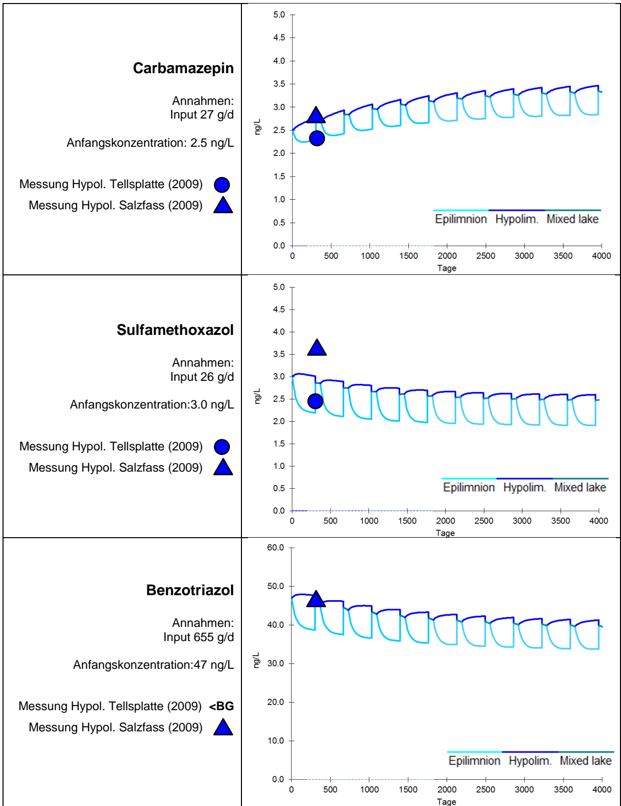
Abbildung 10: Modellierte Konzentrationsverläufe im Vierwaldstättersee für 10 Jahre, ausgehend von der Belastung von 2009 (Messungen Oktober 2009) für die Arzneimittel Carbamazepin und Sulfamethoxazol und das Korrosionsschutzmittel Benzotriazol.
