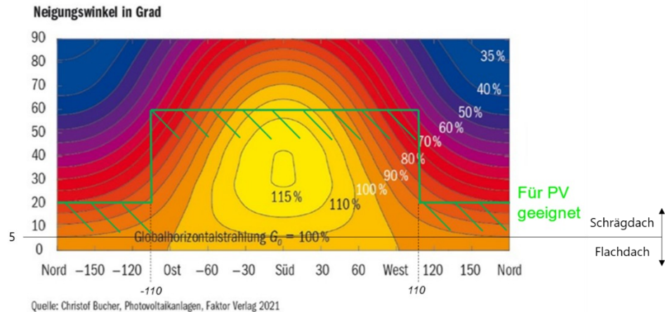
Abbildung 2: Teildachflächen unterhalb der grünen Linie gelten als nutzbare Teildachflächen, sofern sie > 25 m 2 sind.
